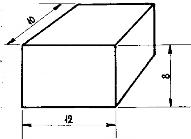
Борова коцка која се користи као подметач кошница при сеоби пчела на паше (Мере изражене у см)
